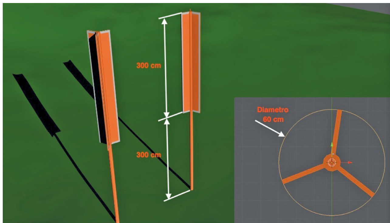
Fig.4.2 Segnale verticale per la segnalazione degli ostacoli agli aeromobili.
